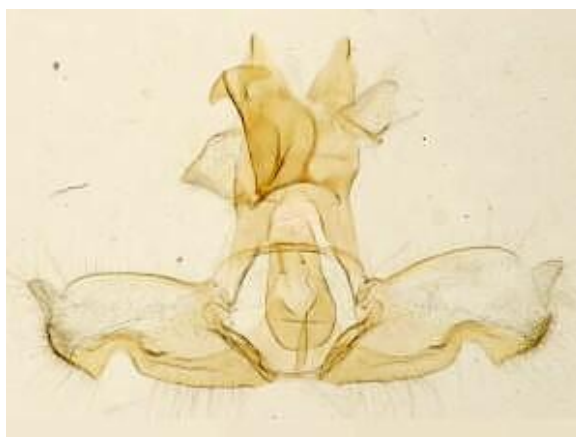
Половой аппарат самца Acleris gloverana ( http://mothphotographersgroup.msstate.edu )
